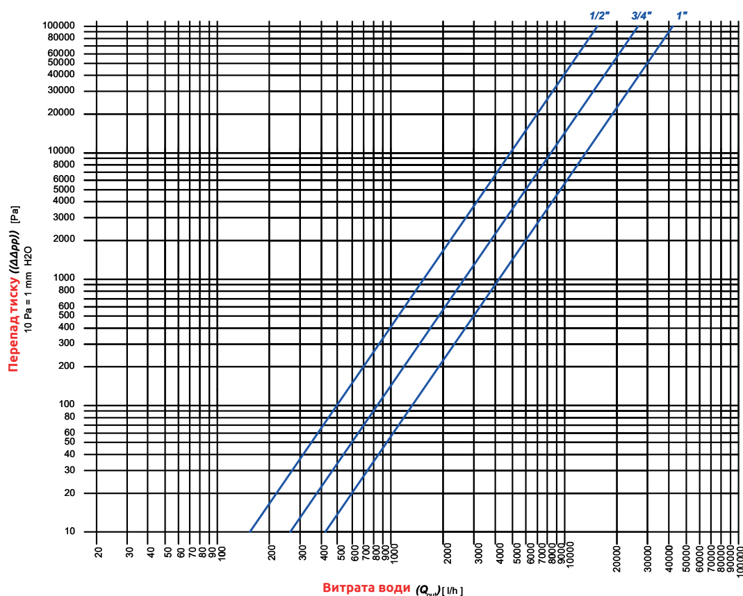
Кульовий кран - Apt. 361 графік перепаду тиску
