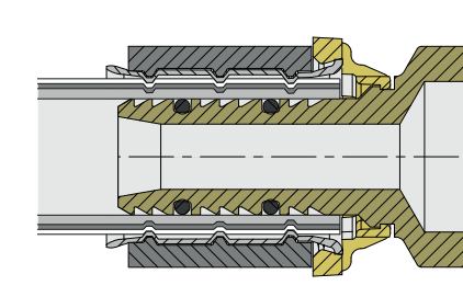
ПРОФИЛЬ U
