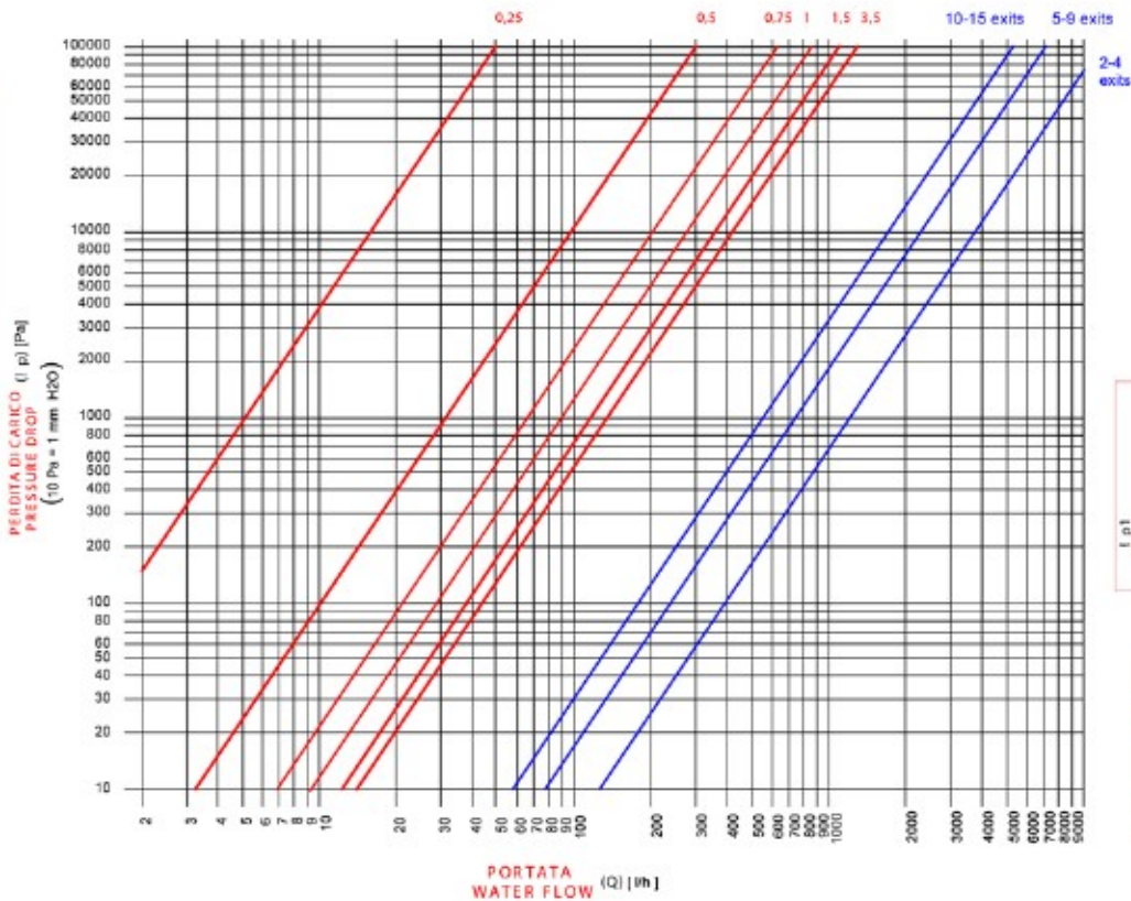
КОЛЕКТОР Арт. 1013-1014-1015-1016 - 1" ДІАГРАМА ВТРАТИ НАВАНТАЖЕННЯ
