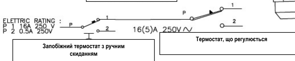
Електрична схема
